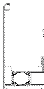
Boční AL profil dvoudílný s přerušným tepelným mostem
