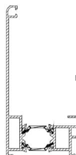
Spodní AL profil jednoduchý s přerušným tepelným mostem
