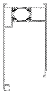
Horní AL profil s přerušným tepelným mostem
